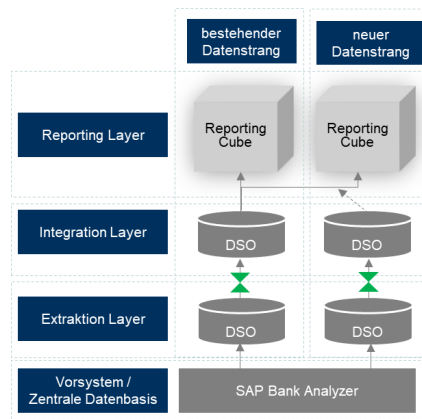
Abbildung 2: Schematische Datenarchitektur
